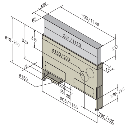
Rückansicht
