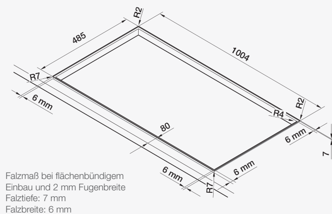
Flächenbündiger Einbau
